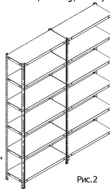
Установка промеж. угловых полок
